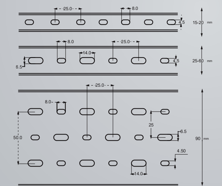
پانچ کف داکت ها مطابق با استاندارد ۵۰۰۸۵ اروپا
